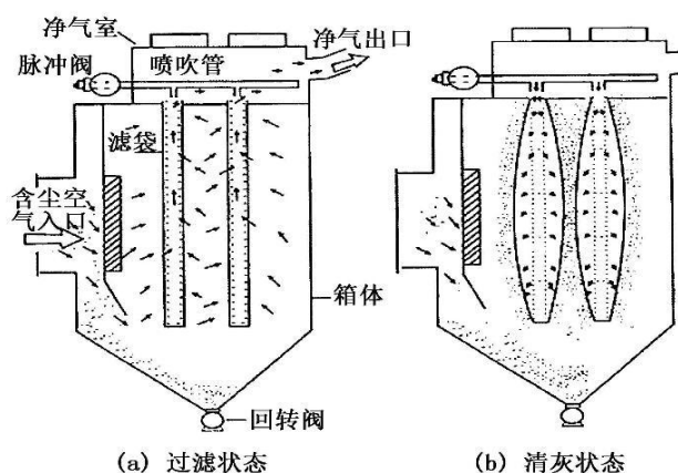
图 4.3-1 脉冲布袋除尘设施处理工艺流程图
