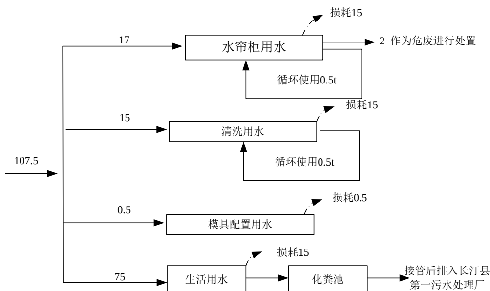
图 2.1-4 全厂给排水平衡图 单位：m 3 /a
