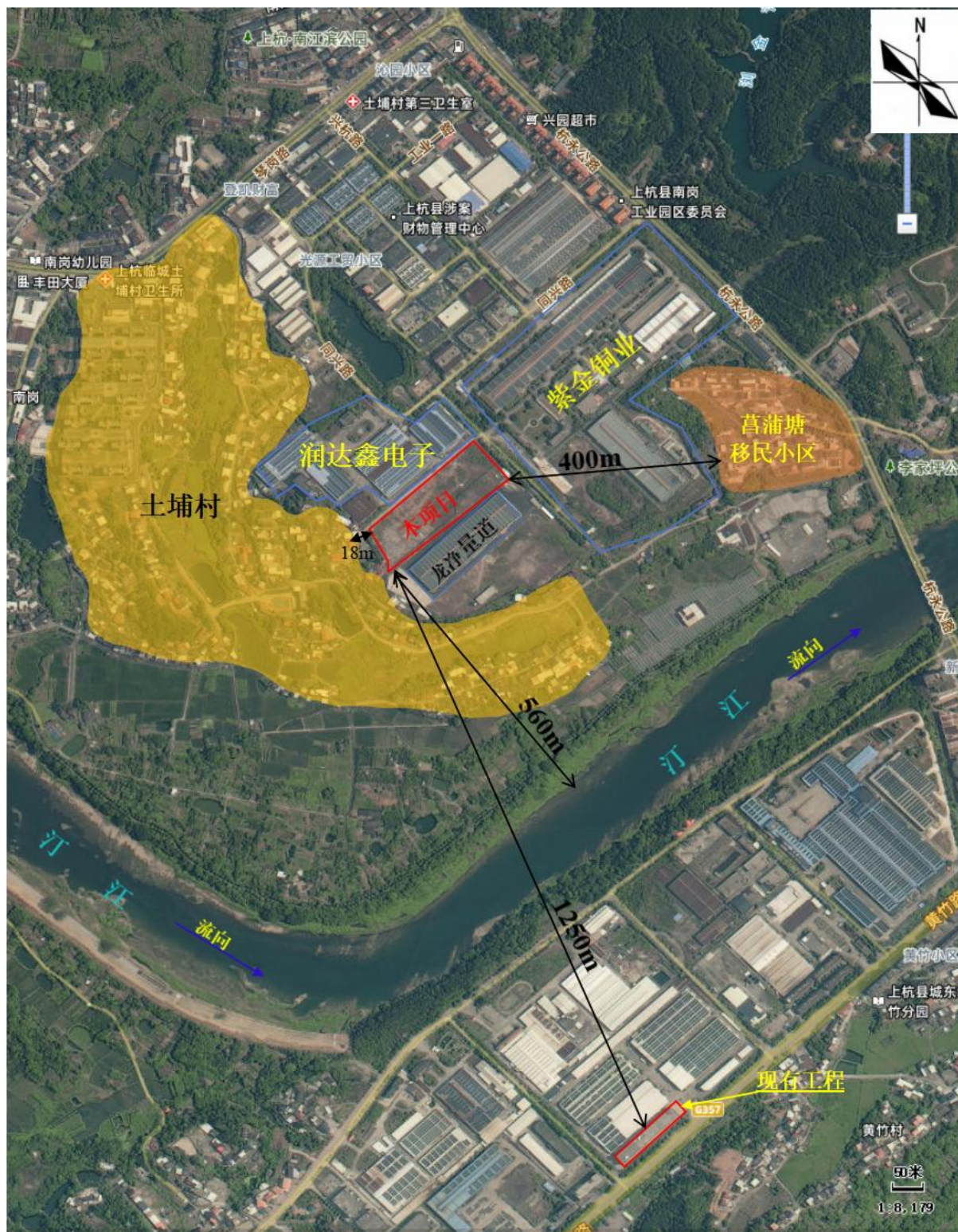
附图3 环境保护目标及周边环境示意图
